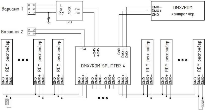
Рис.2 – Схема подключения изделия
