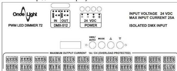
Рисунок 2. Внешний вид лицевой панели прибора
