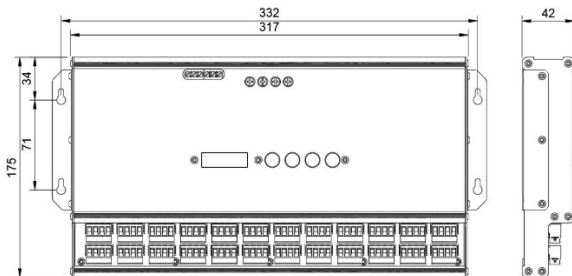
Рисунок 1. Внешний вид и габариты
