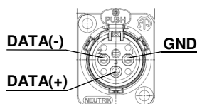
Рис.2 – Цоколёвка DMX OUT
