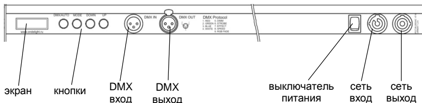
Рис.4 – Вид сзади
