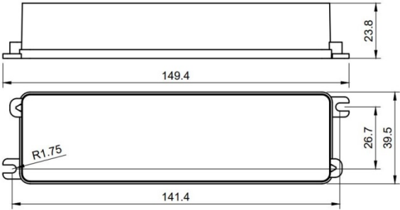
Рисунок 1 – Внешний вид и габариты диммера
