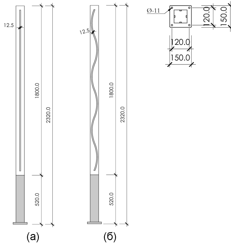
Рисунок 1. Внешний вид и габариты светильников BWL(а) и BWW(б)
