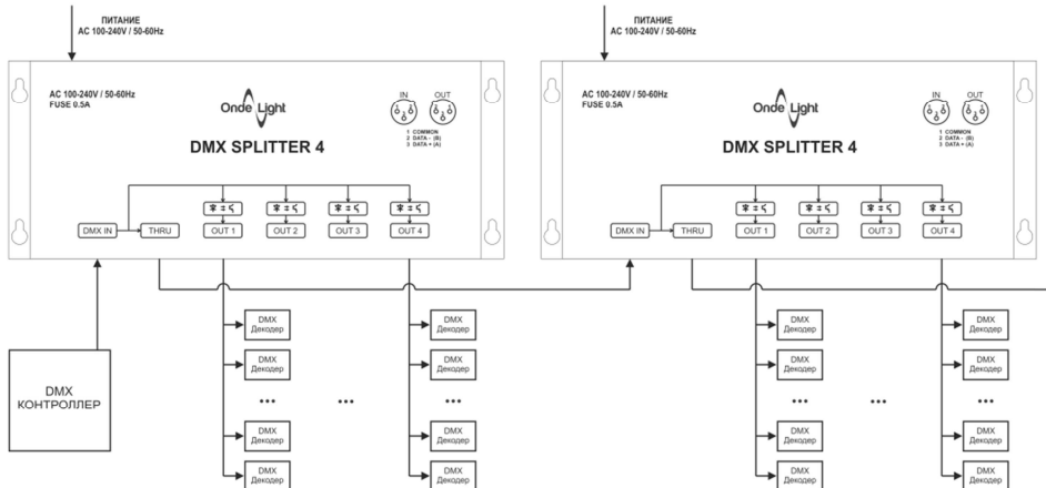
Рис.2 – Схема подключения изделия
