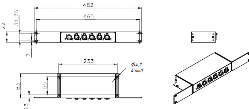
Рис.1 – Внешний вид и размеры
