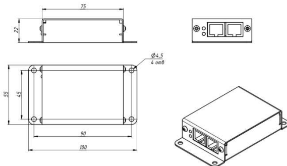
Рисунок 1 – Внешний вид и габариты диммера
