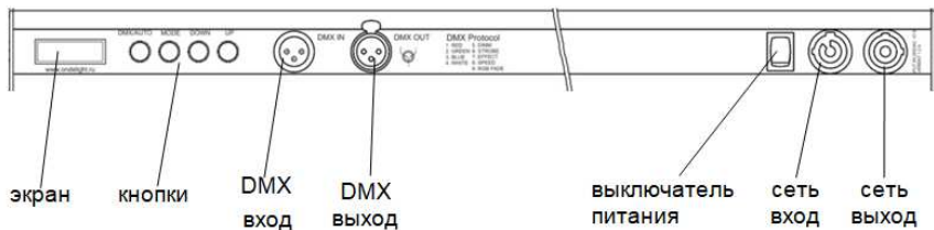
Рис.2 Внешний вид задней панели прожектора и основные органы управления
