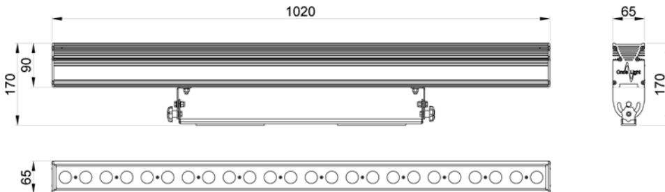
Рис.1 – Внешний вид и габаритные размеры
