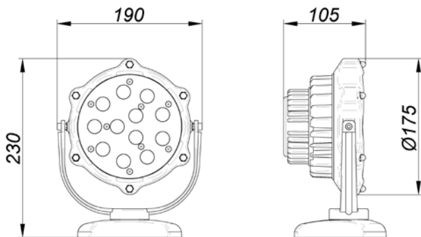
Рис.1 – Внешний вид и размеры
